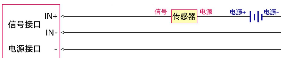
二线制电流信号采集单端接线图
