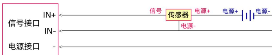
三线制电流信号采集单端接线图
