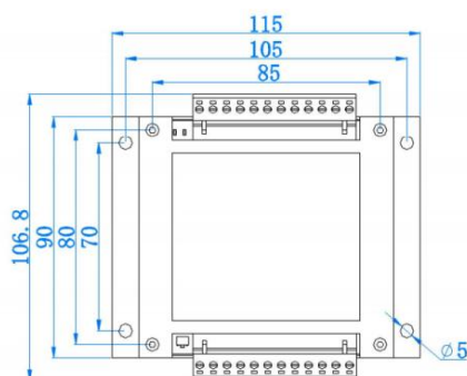
主视图
