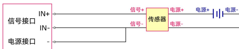
电压信号采集单端接线图
