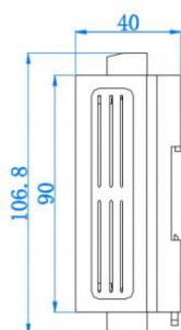
右视图
