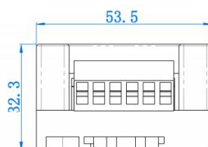
仰视图
