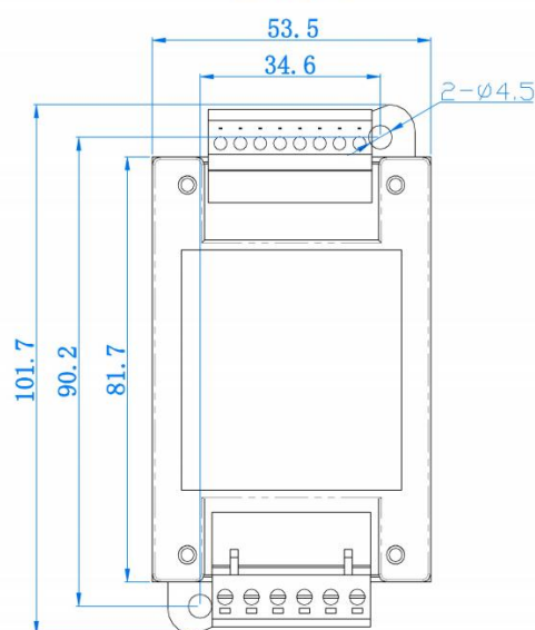
主视图
