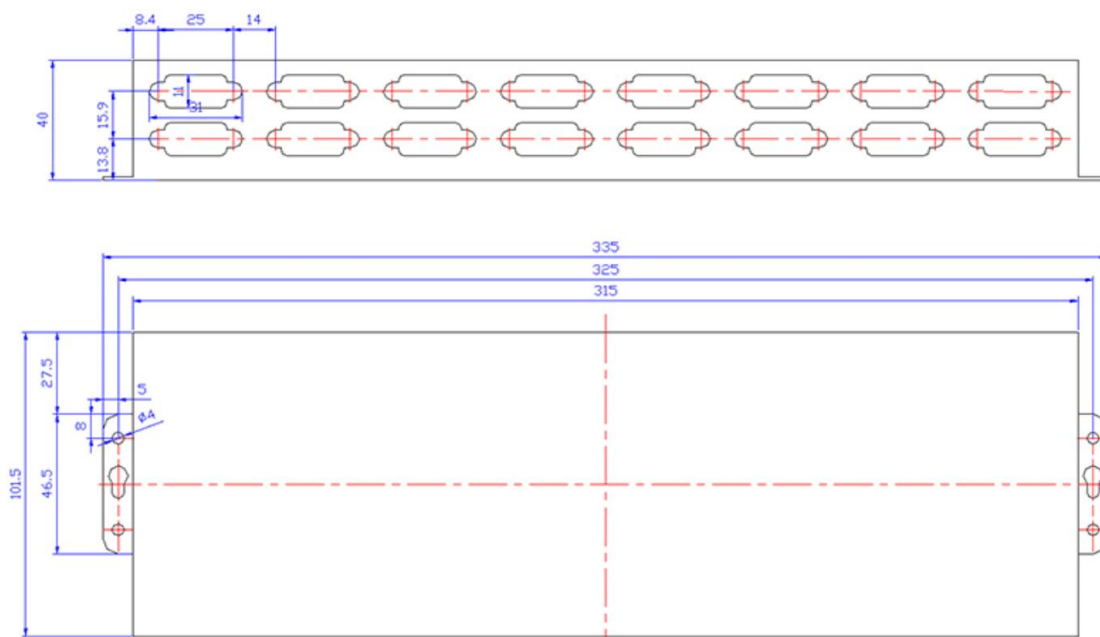
侧面图
