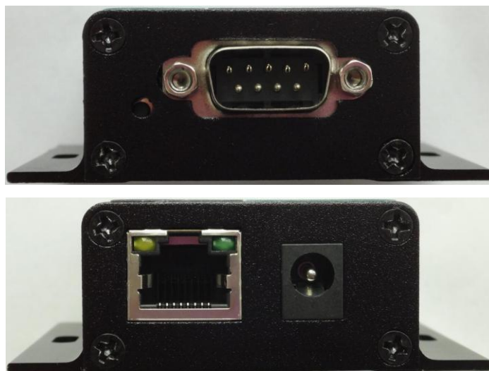
图 1 模块接口
