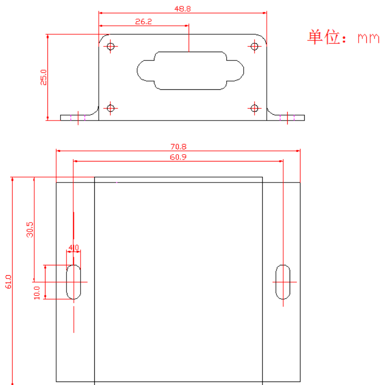
图 2 尺寸
