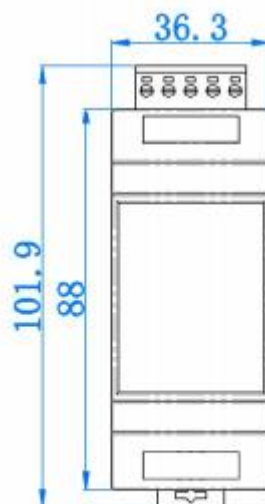
主视图
