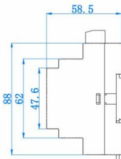
右视图
