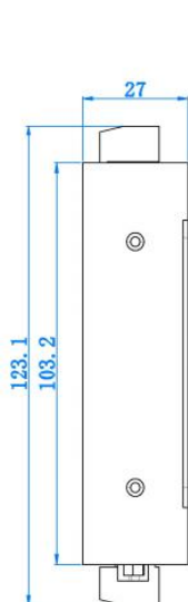
右视图
