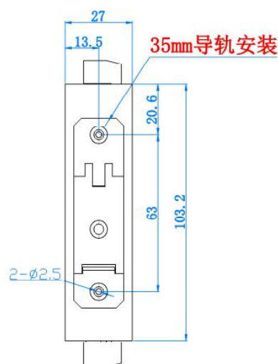
左视图
