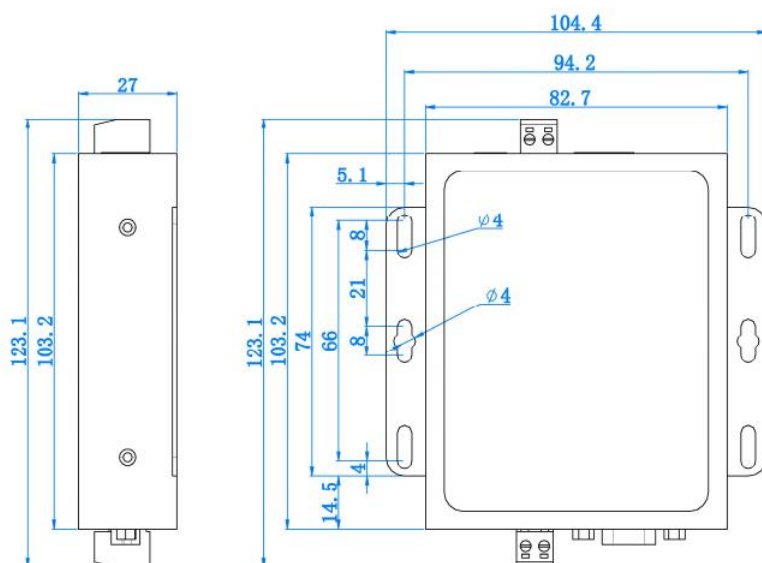
右视图
