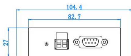
仰视图
