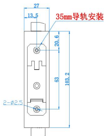
左视图
