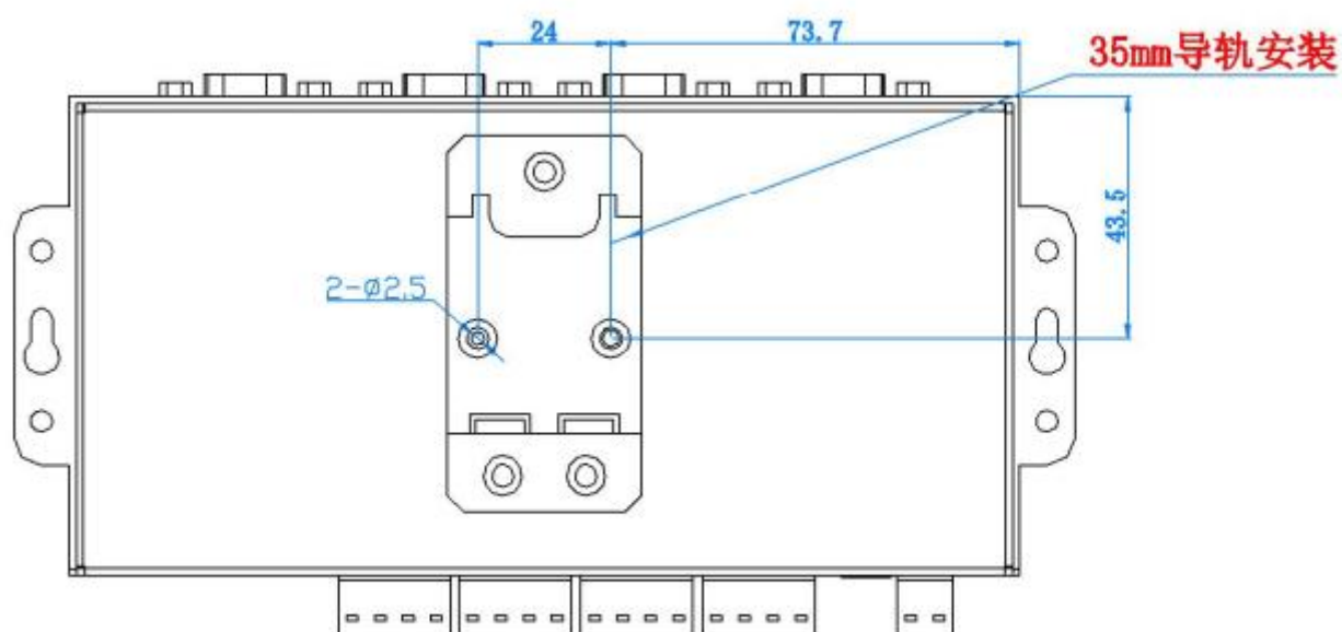
后视图
