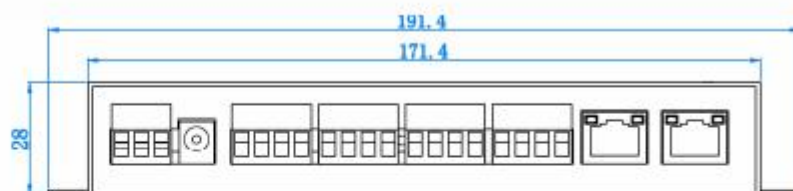
仰视图
