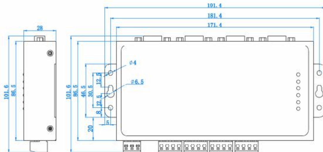
右视图
