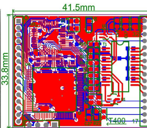
图 2 PCB 尺寸
