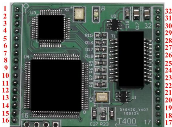
图 3 管脚位置
