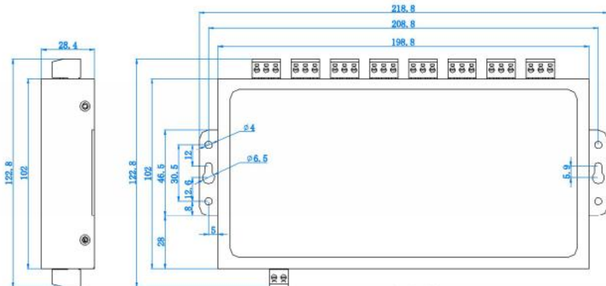
右视图
