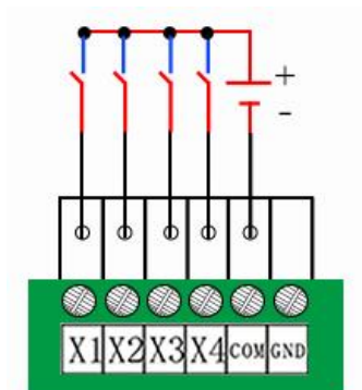
图 4.8 湿节点接法
