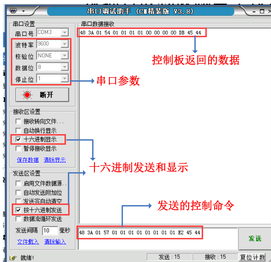
图 2.5 串口调试助手发送控制指令
