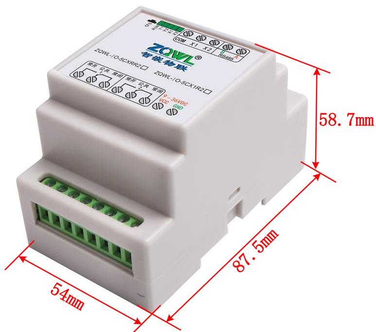
图 4.4 设备机械尺寸 1
