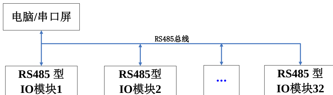
图 6.1 IO 设备与 RS485 IO 设备级联
