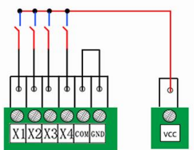
图 4.7 干节点接法
