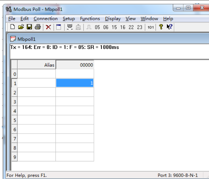
图 2.8 Modbus poll 控制继电器
