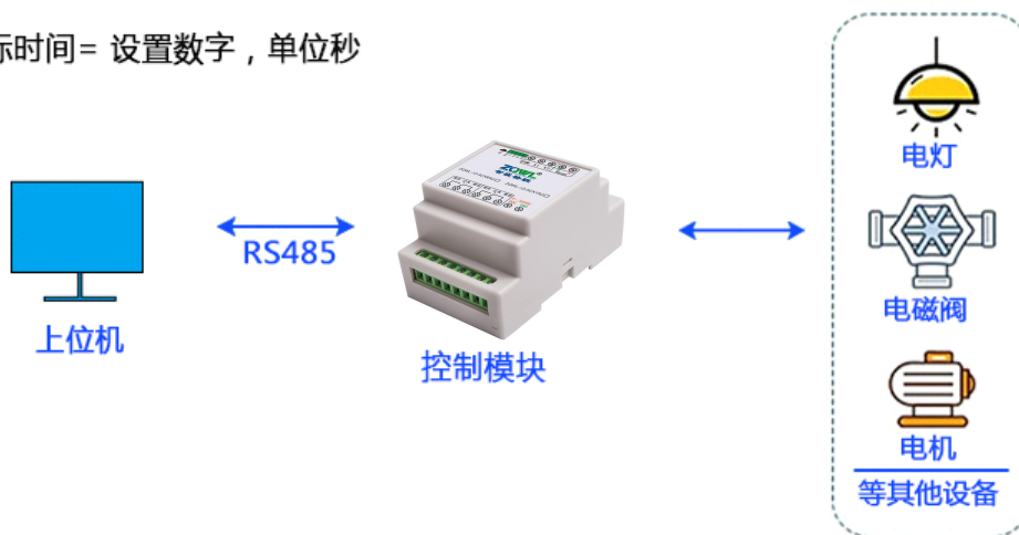
图 6.5 延时断开控制
