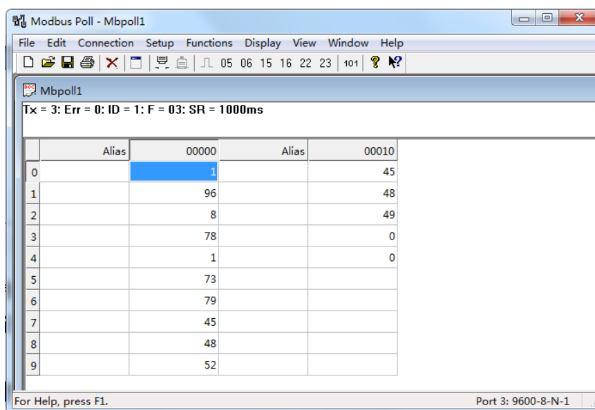
图 2.6 Modbus poll 读设备信息
