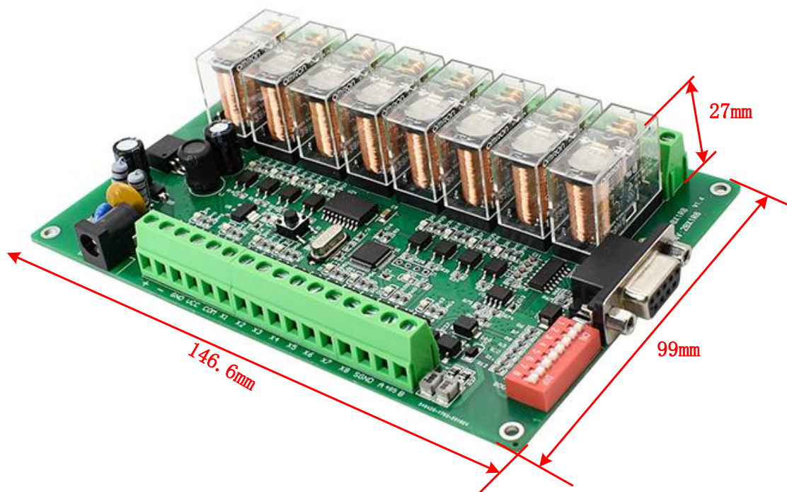
图 4.3 设备的接口布局 2
