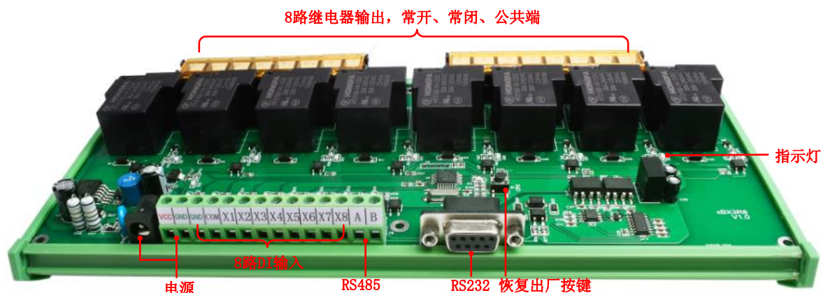
图 4.11 设备的接口布局 6
