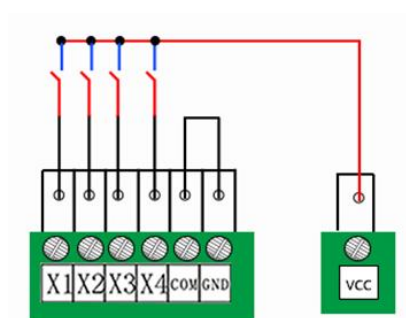
图 4.15 干节点接法
