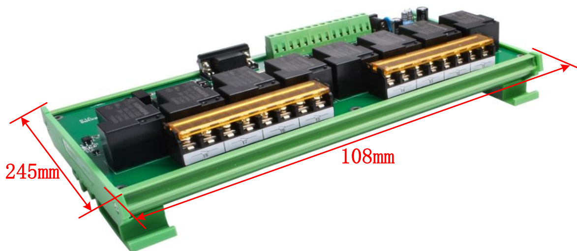
图 4.11 设备的接口布局 6
