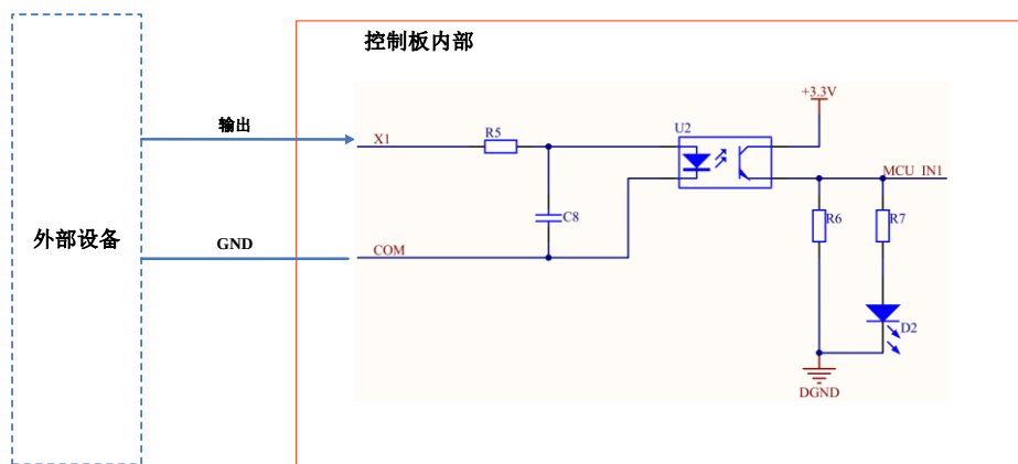
图 4.13 PNP 接线方式
