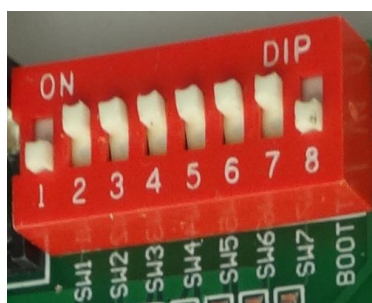
图 4.17 拨码开关
