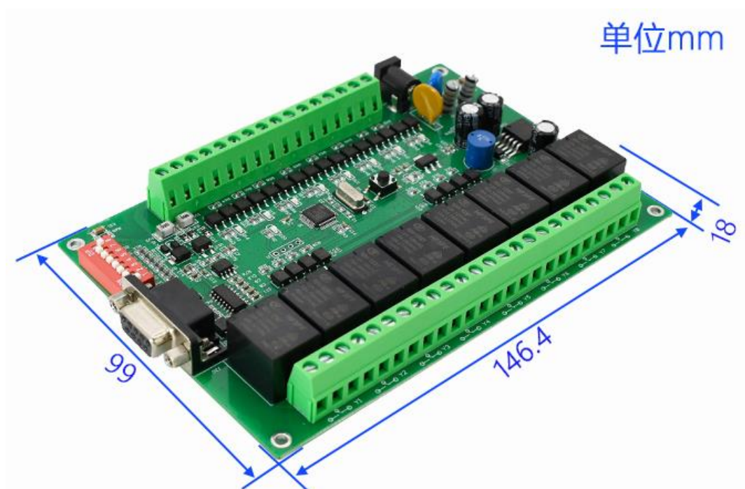
图 4.2 设备机械尺寸 1
