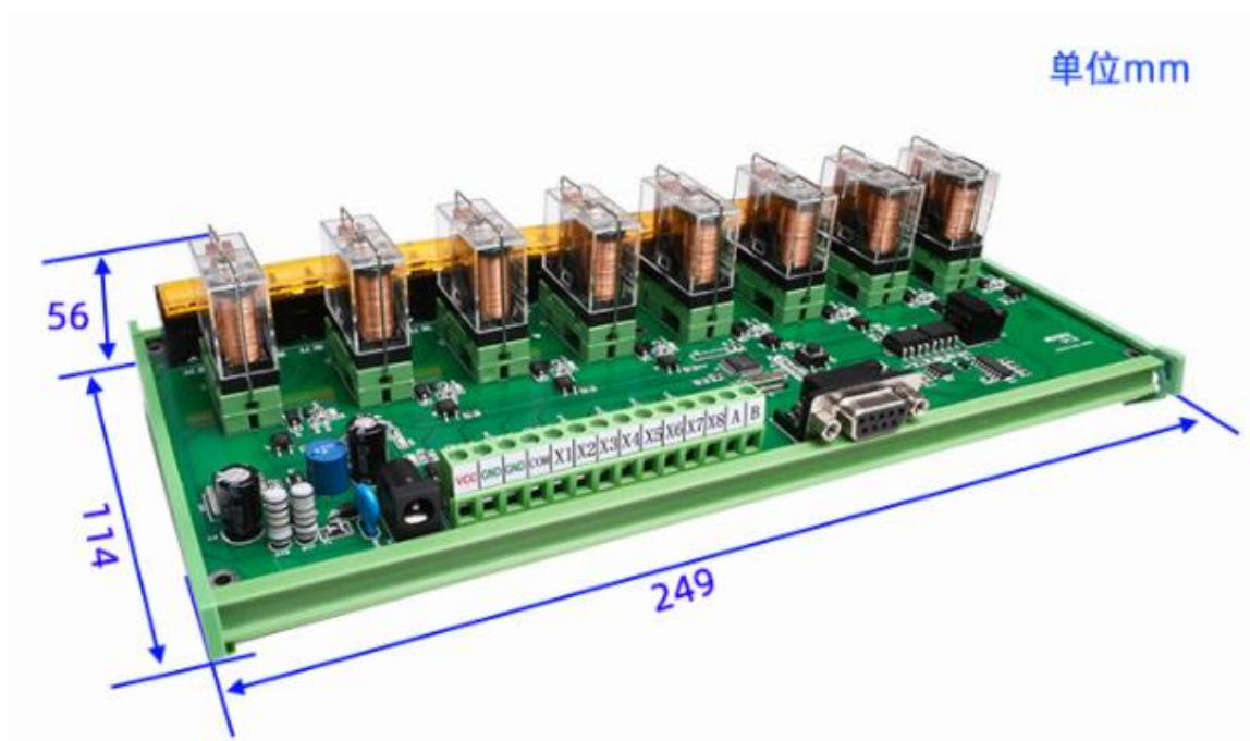
图 4.10 设备机械尺寸 5
