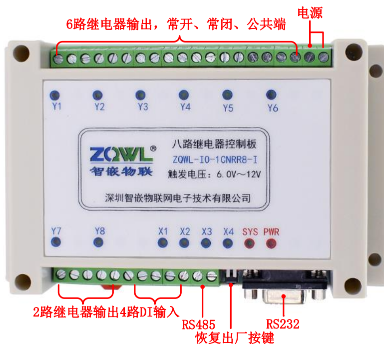
图 4.5 设备的接口布局 3
