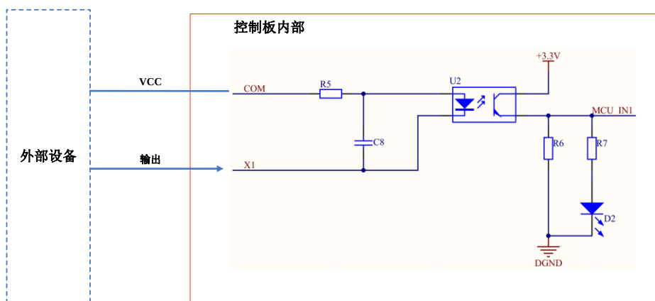
图 4.14 NPN 接线方式
