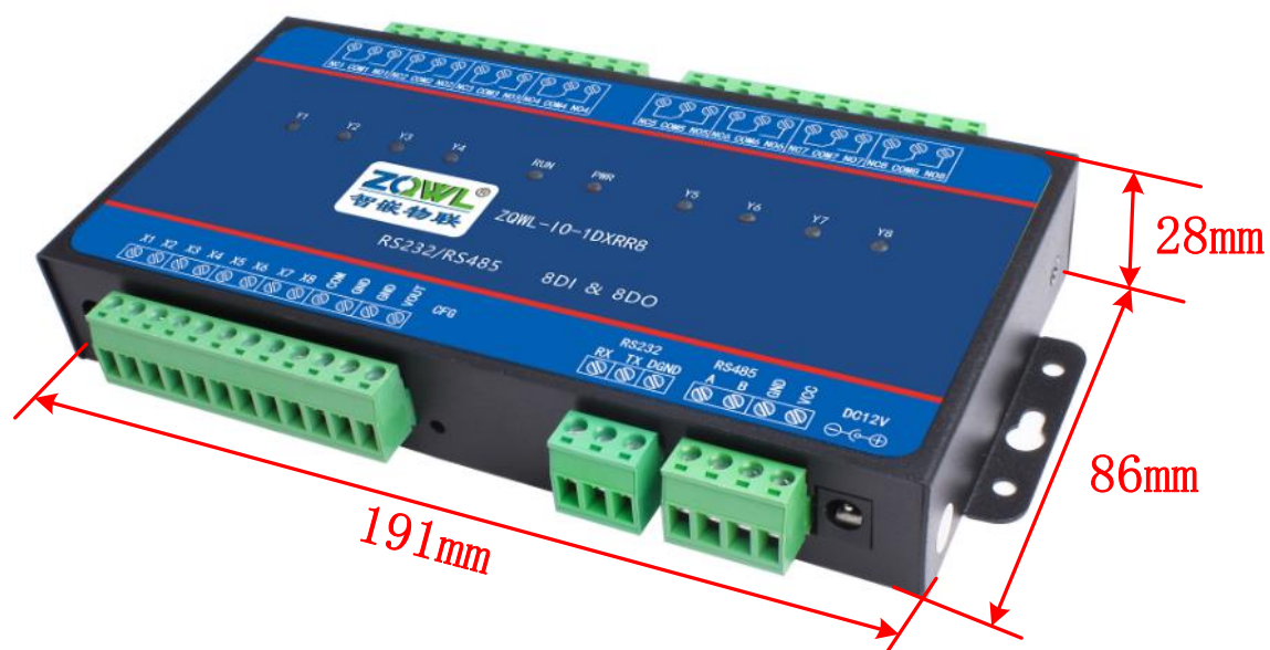
图 4.8 设备机械尺寸 4
