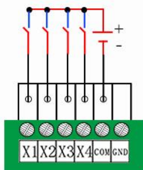
图 4.16 湿节点接法
