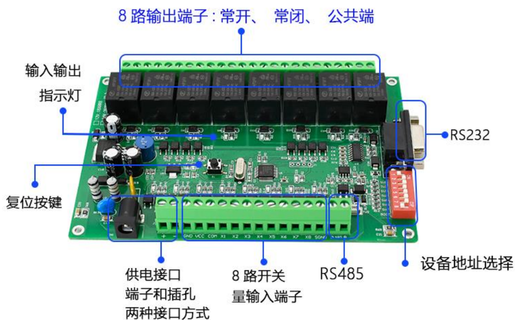
图 4.1 设备的接口布局 1
