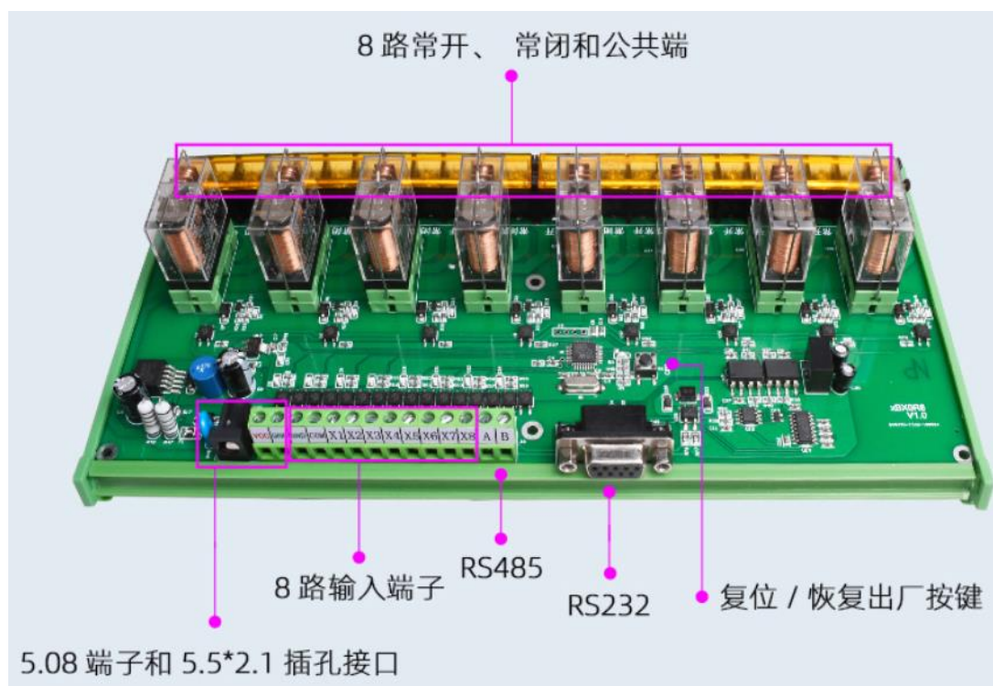
图 4.9 设备的接口布局 5
