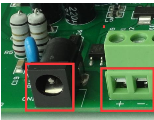
图 2.2 电源接口
