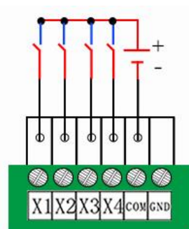
图 4.8 湿节点接法
