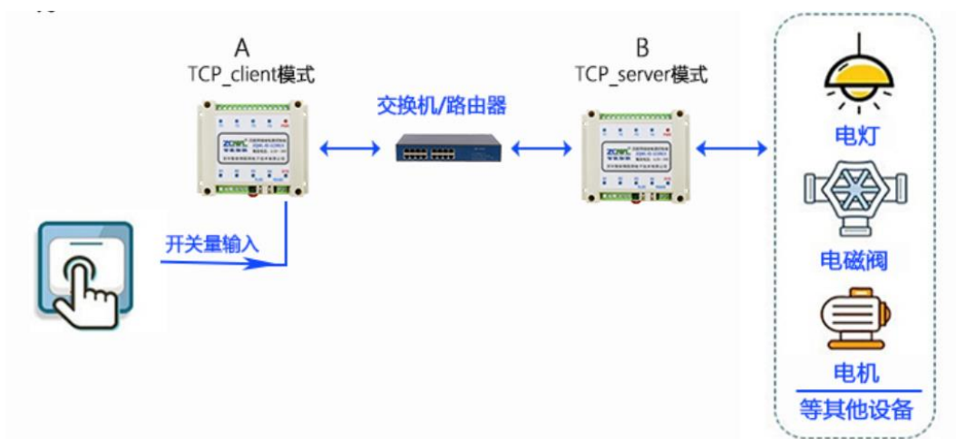
图 6.4 设备间联动
