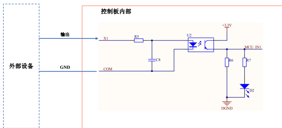
图 4.5 PNP 接线方式
