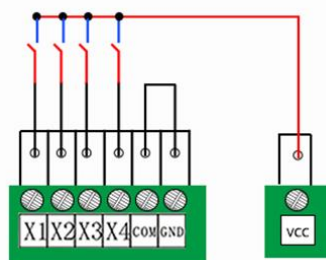
图 4.7 干节点接法
