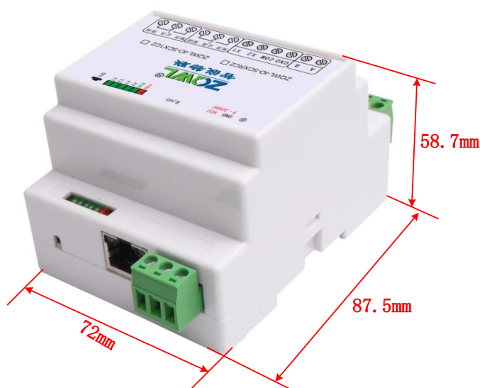
图 4.2 设备机械尺寸 1
