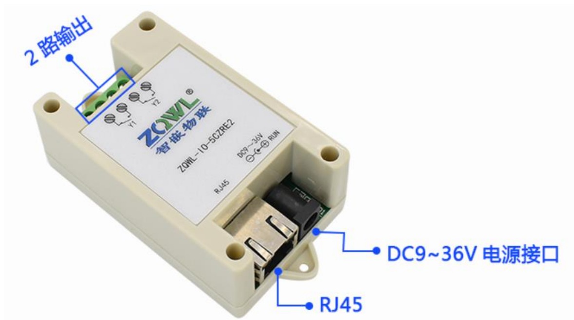
图 4.3 设备的接口布局 2
