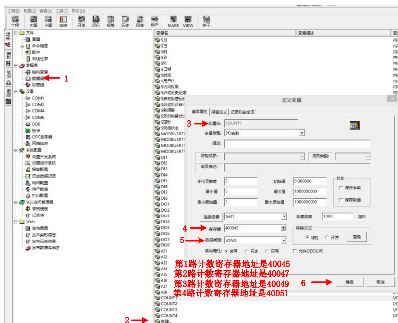
图 9.25 组态王添加脉冲计数变量
