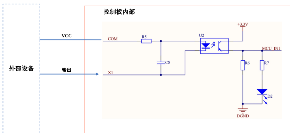
图 4.6 NPN 接线方式
