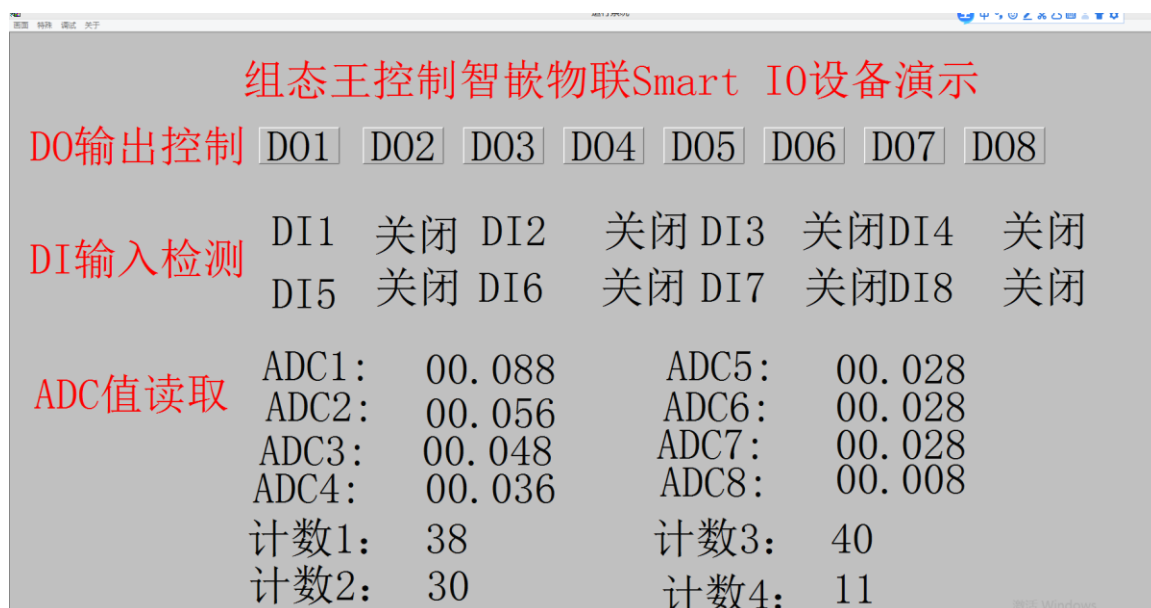
图 9.32 组态王软件读取 Smart IO 设备数据
