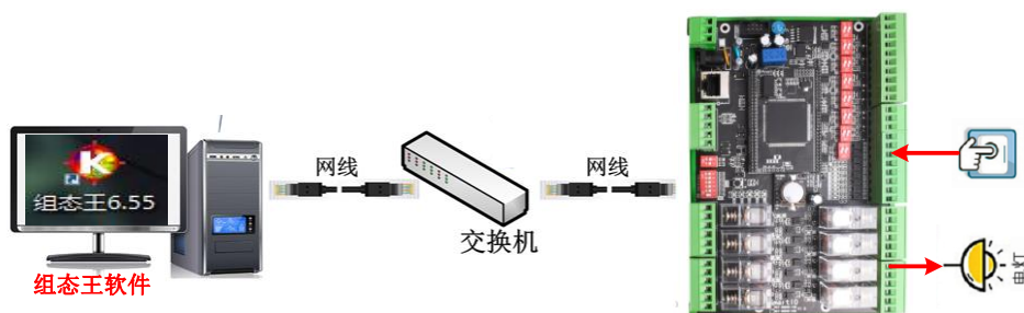
图 9.16 设备与组态王通信硬件连接
