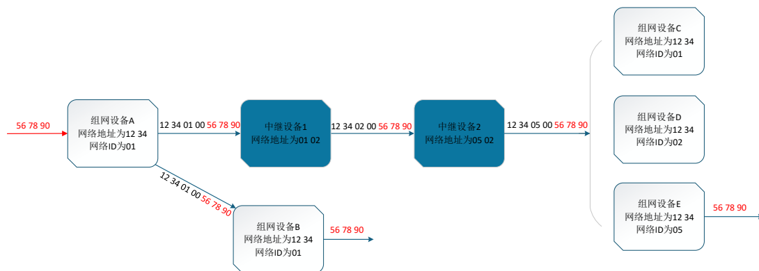
图 6-15 中继原理
