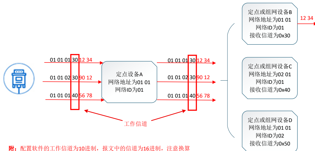
图 6-11 定点模式
