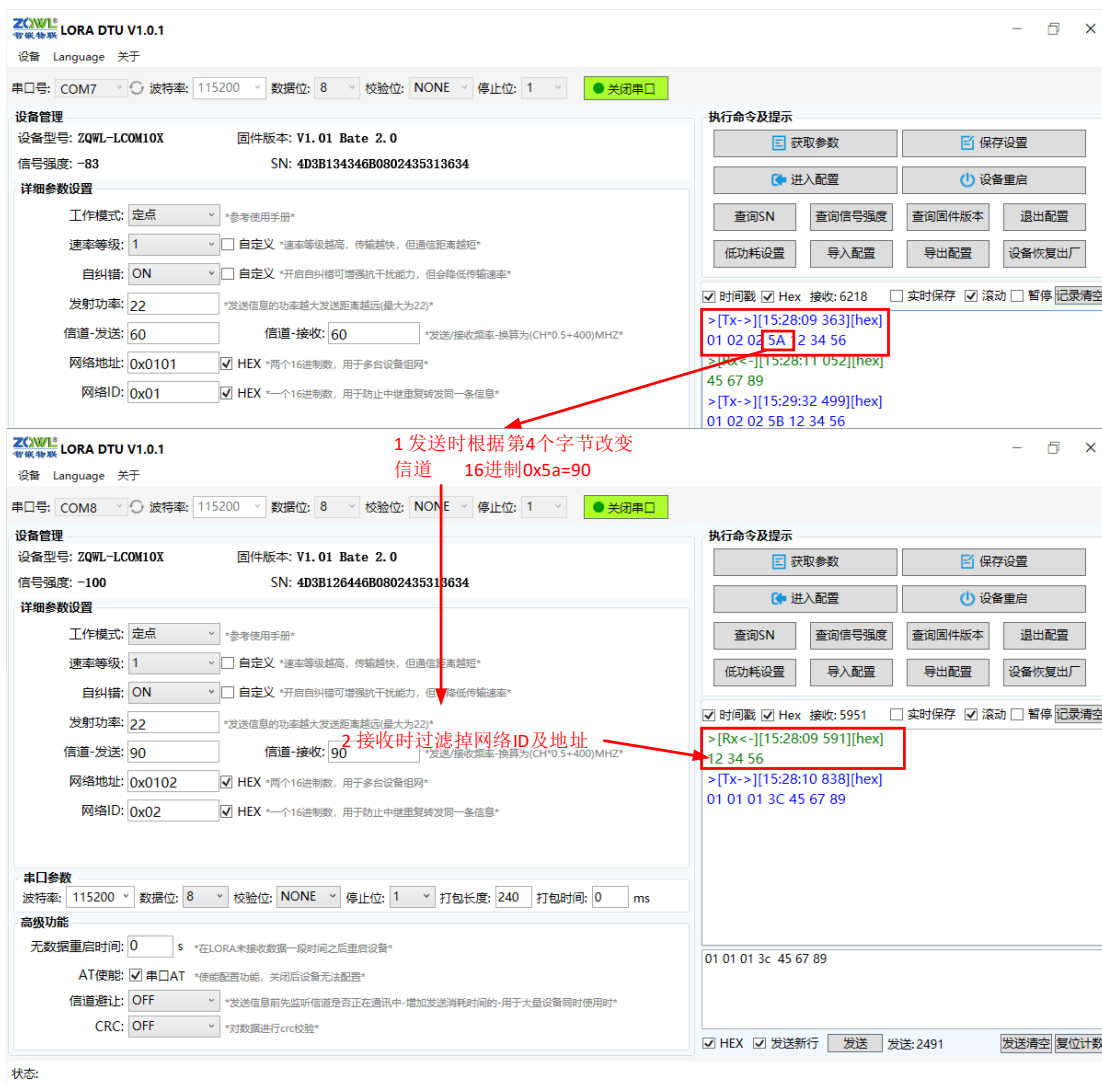
图 6-14 定点与定点通讯
