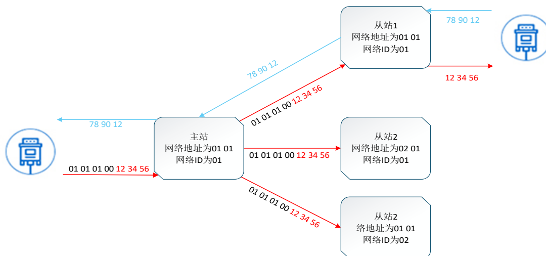
图 6-7 主站从站
