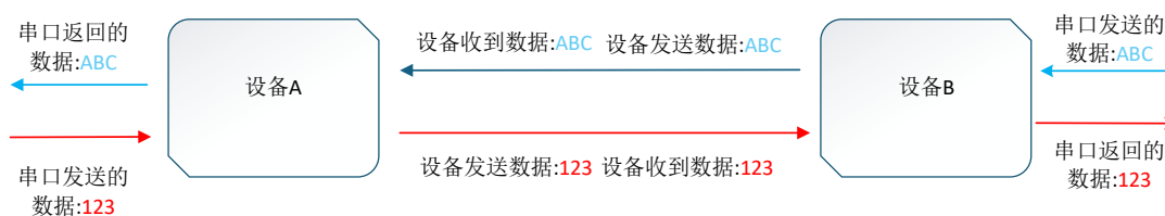
图 6-1 透传模式
