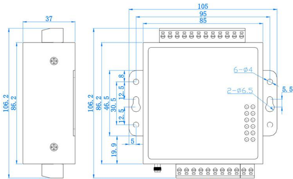
右视图
