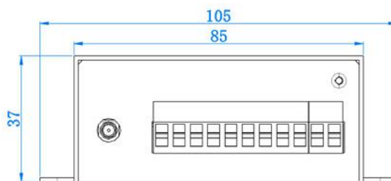
仰视图
