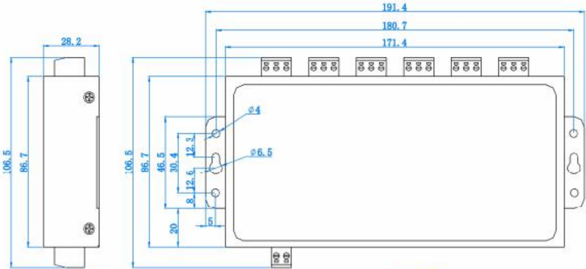
右视图
