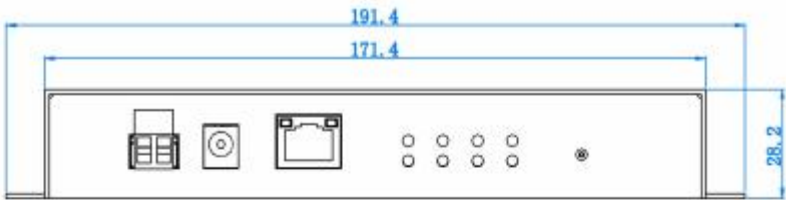
仰视图
