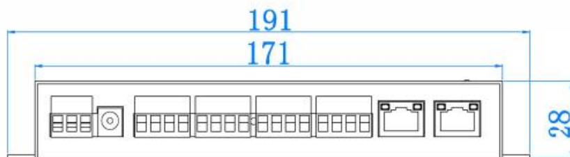
仰视图
