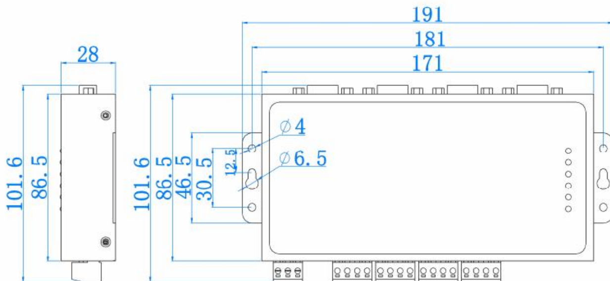
右视图
