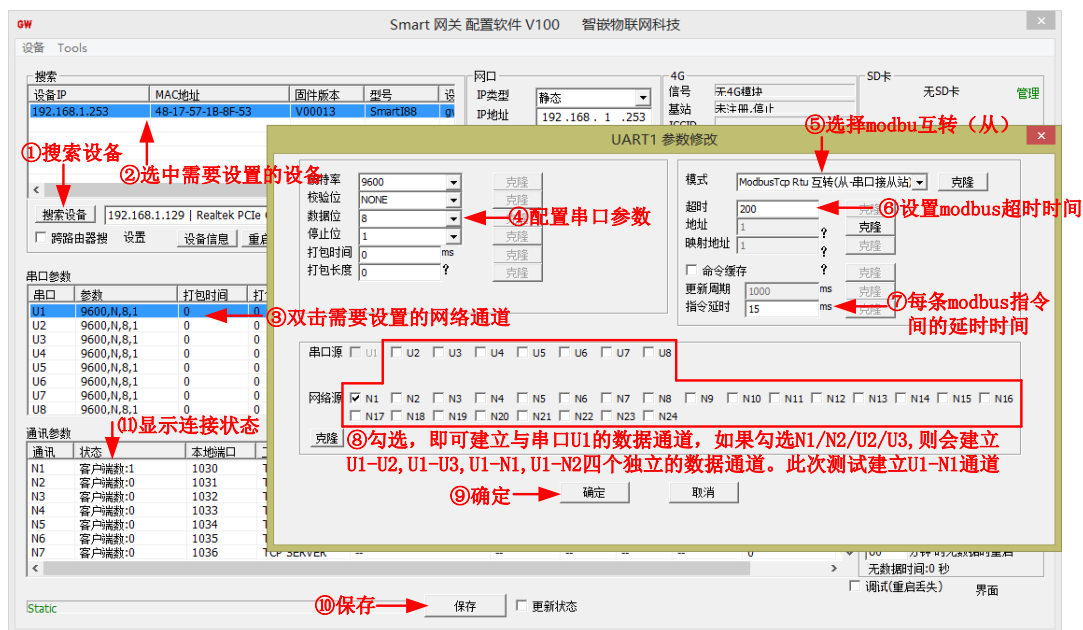
图 3.23 ModBus TCP/RTU 互转（从）模式配置
