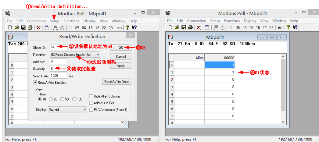
图 4.25 读取 8 路 DI 状态
