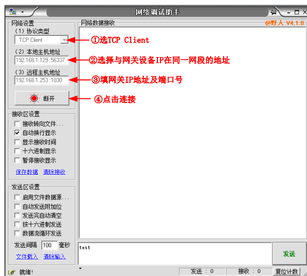
图 2.8 网络调试助手参数设置
