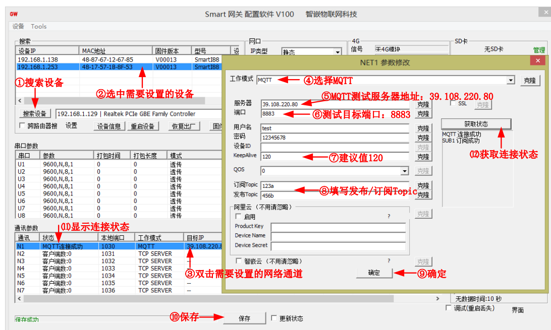
图 4.9 N1 通道配置为 MQTT 模式
