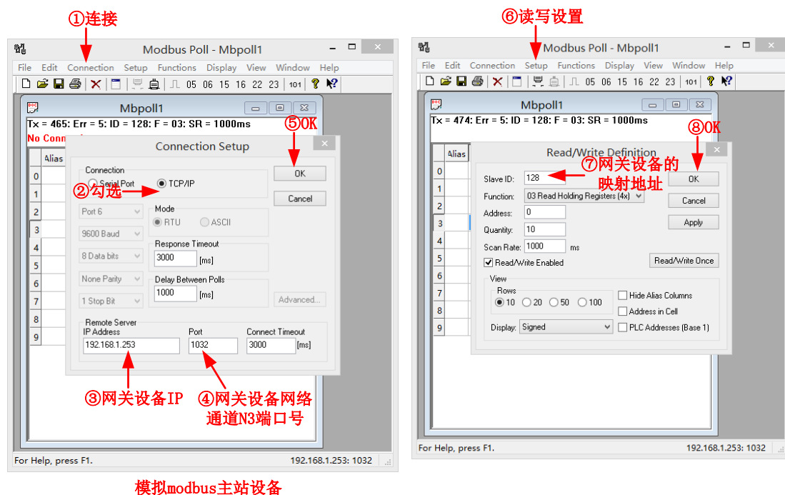
图 7.11 配置 Modbus Poll
