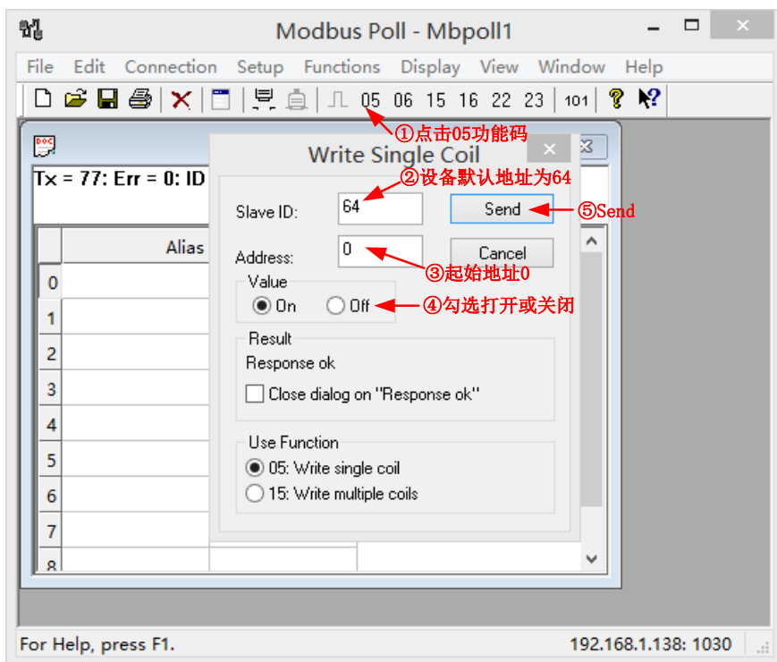
图 4.26 控制单路 DO 输出
