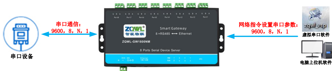
图 5.7 自设波特率原理框图
