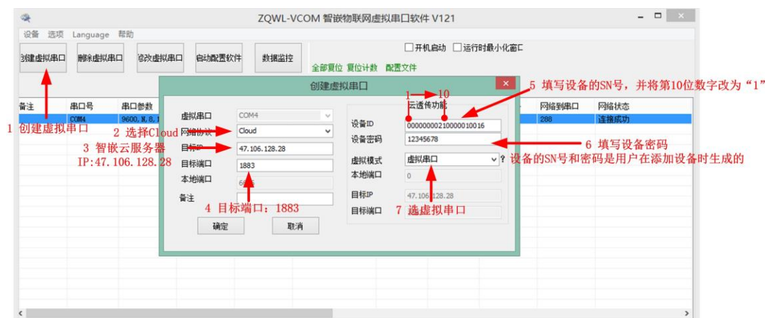
图 4.22 虚拟串口接入智嵌云并绑定设备步骤
