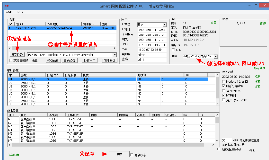
图 4.17 智嵌云参数配置 1
