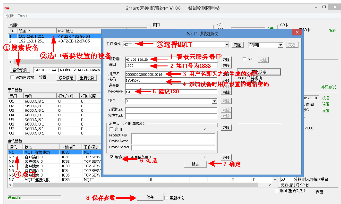
图 4.18 智嵌云参数配置 2
