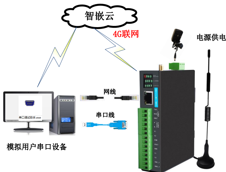
图 4.8 远程采集串口设备数据示意图
