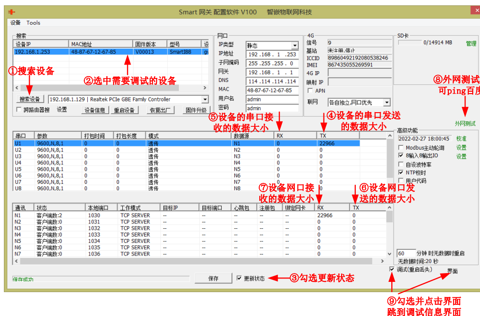
图 5.13 调试界面 1
