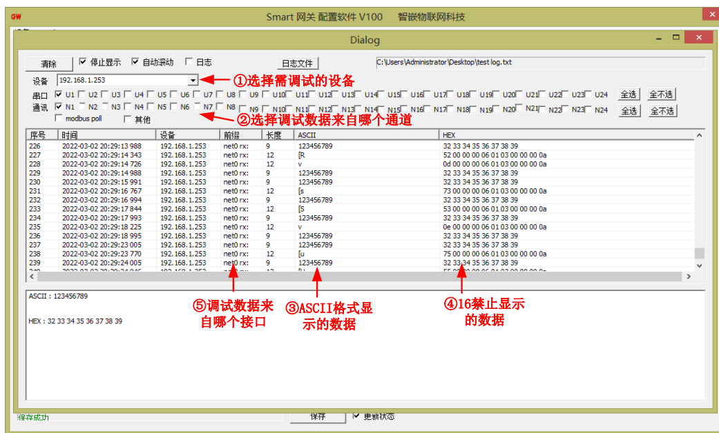
图 5.14 调试界面 2
