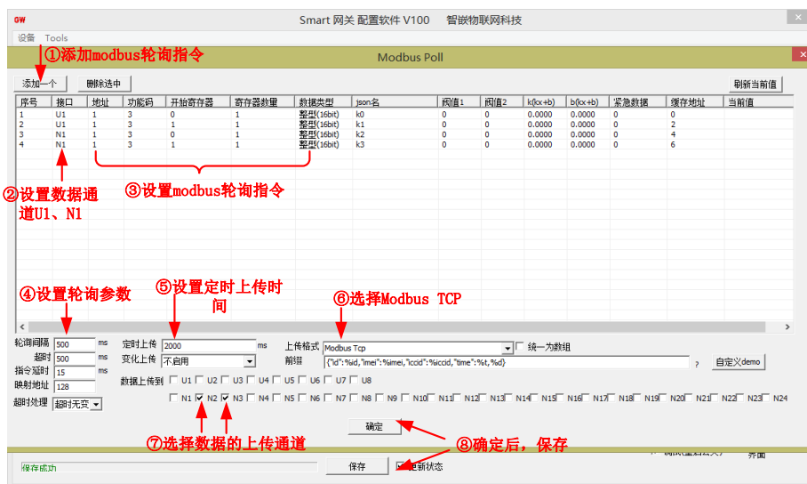
图 7.6 轮询通道 U1、N1 并上传到 N2、N3 通道
