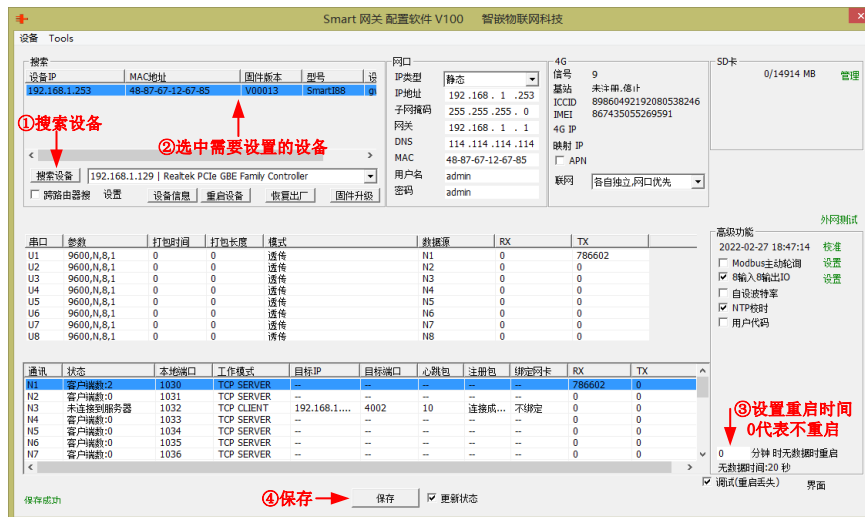
图 5.6 无数据重启配置
