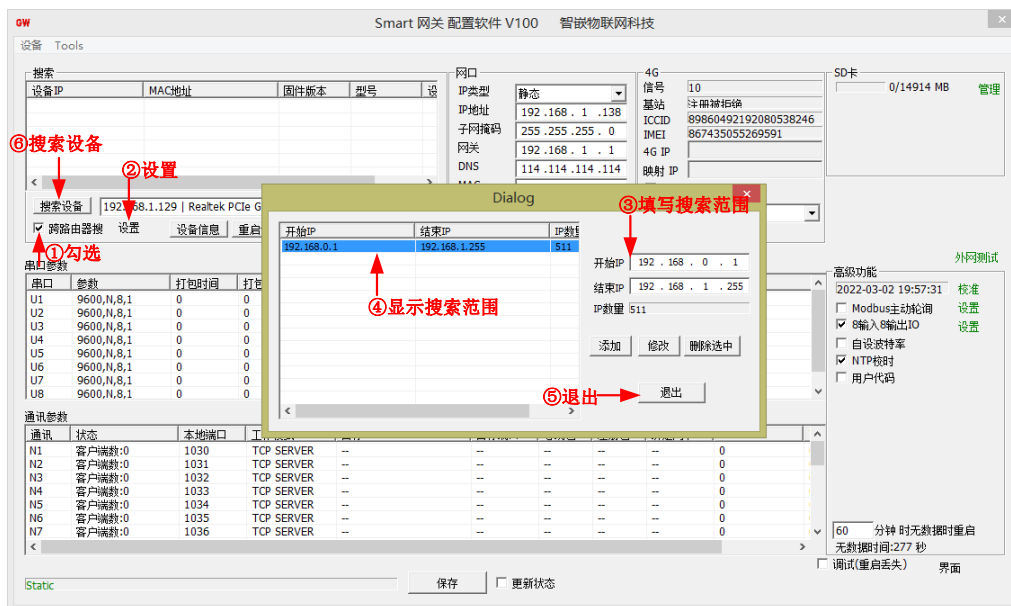
图 5.10 跨路由搜索配置
