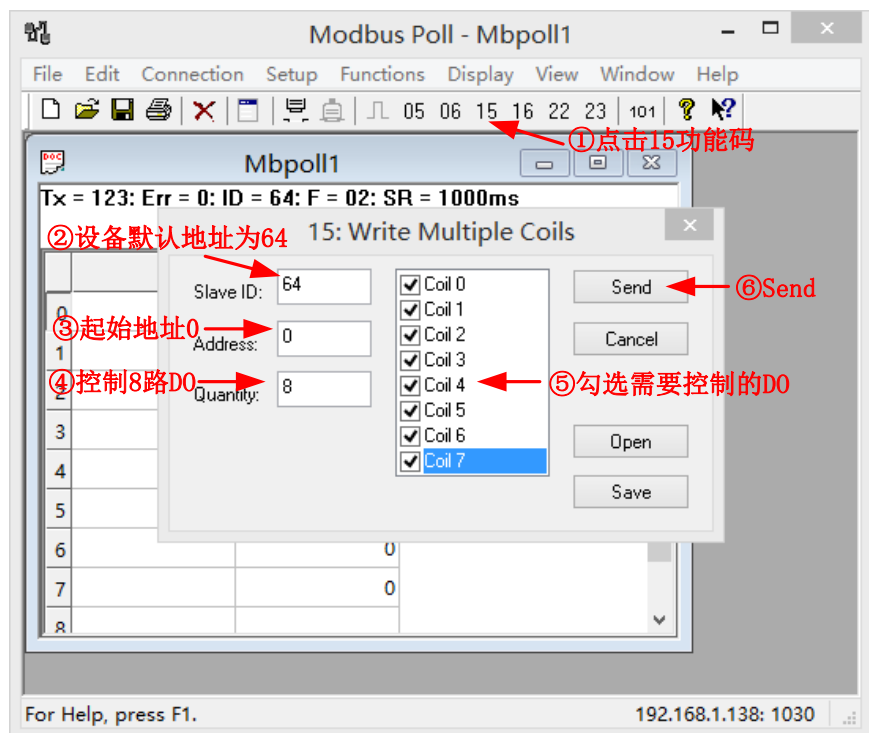
图 4.27 控制多路 DO 输出
