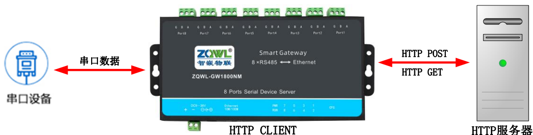
图 3.13 HTTP POST/GET
