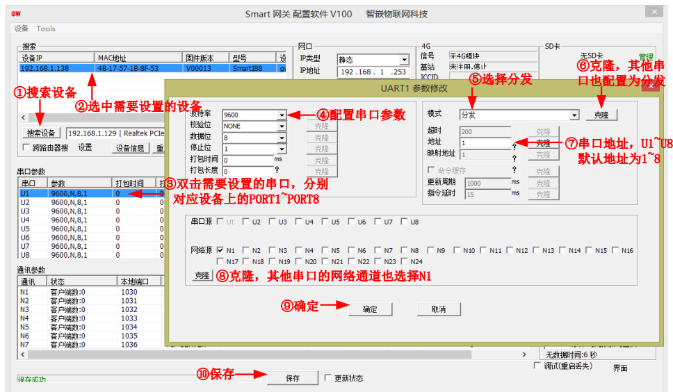
图 3.34 分发配置
