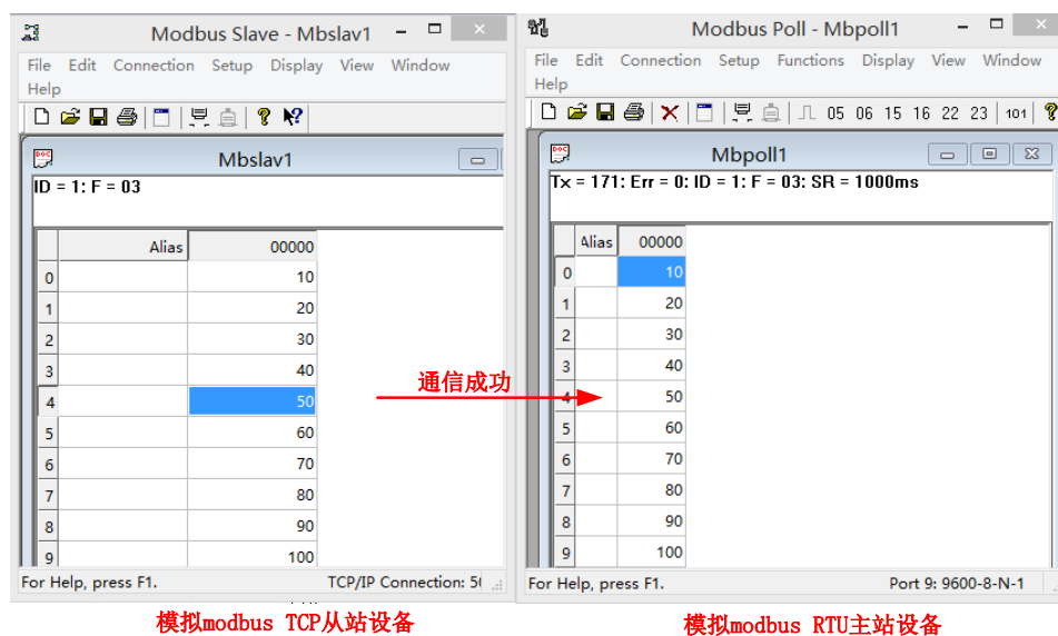
图 3.30 通信成功
