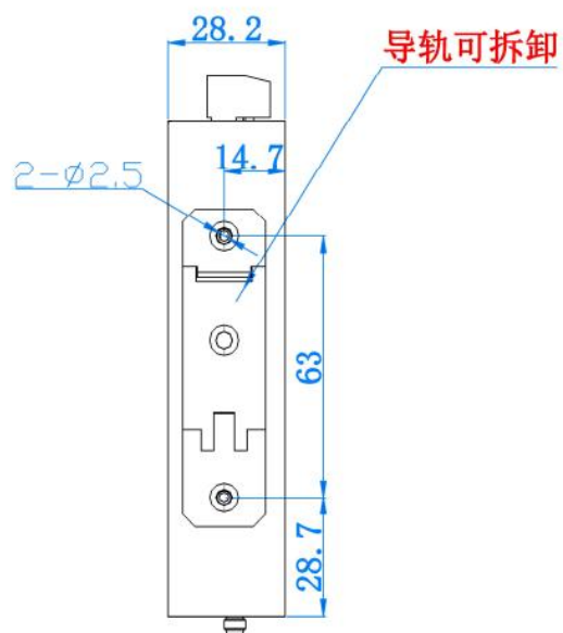
左视图
