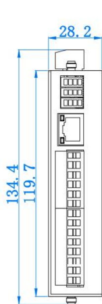
右视图
